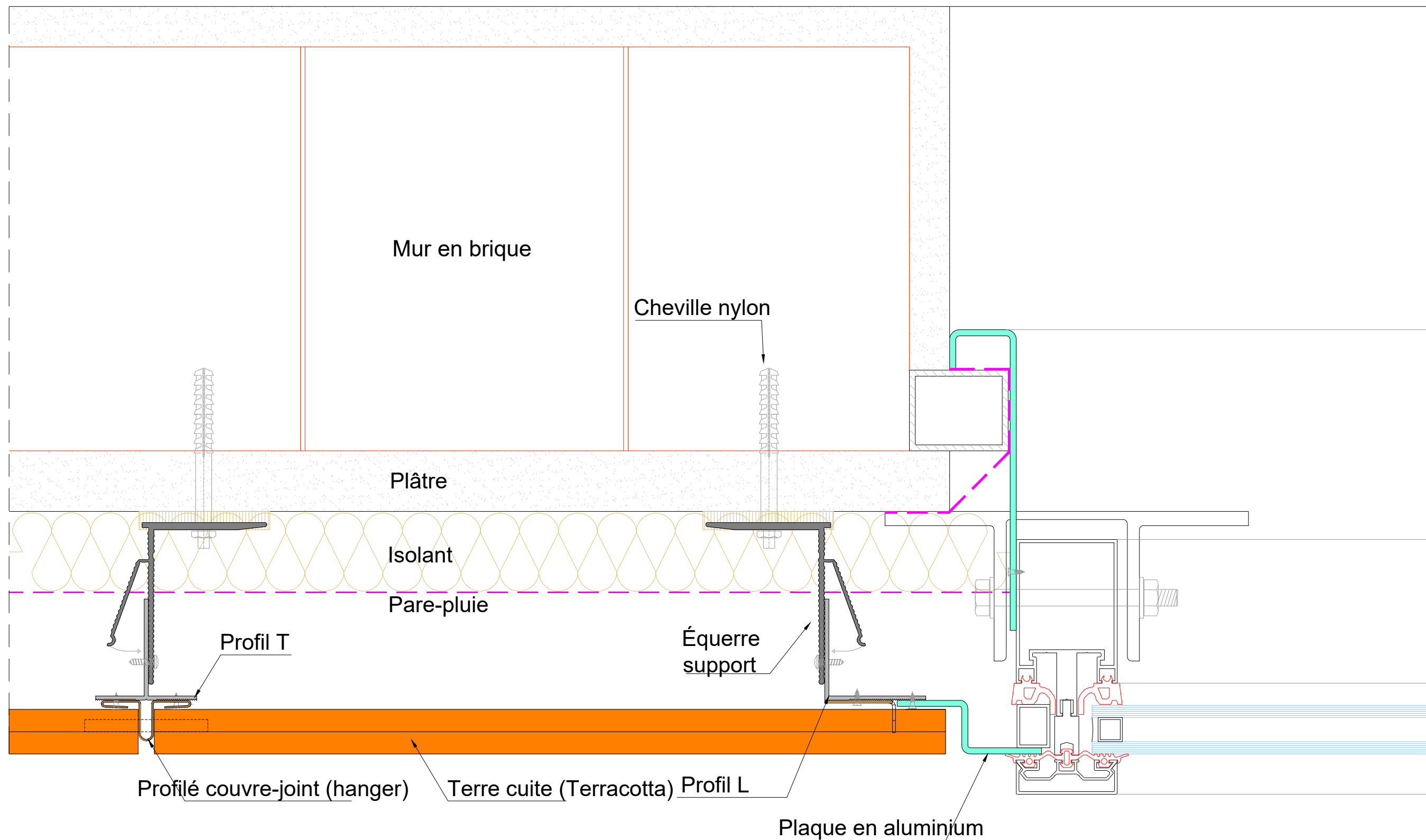
DÉTAIL A
